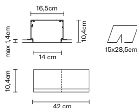
CASSAFORMA 14x28 cm / WALLBOX 14x28 cm
