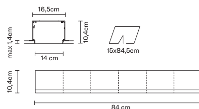
CASSAFORMA 14x84 cm / WALLBOX 14x84 cm
